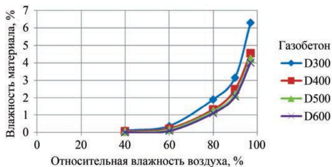
Рис. 1. Изотермы сорбции образцов газобетона
